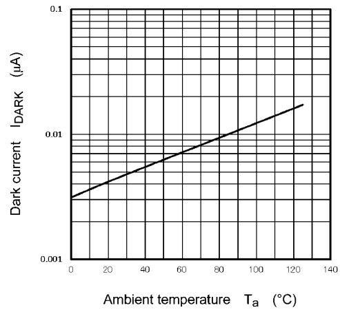
Fig. 11.10 I_{DARK} - T_a
