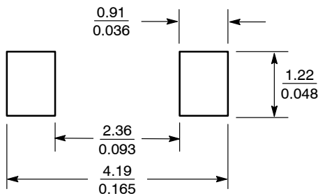
SCALE 10:1 \left(\frac{\text{mm}}{\text{inches}}\right)
